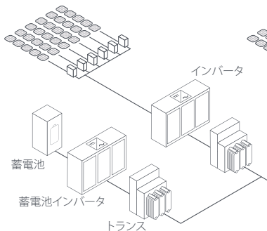
AC側接続の蓄電池システム
