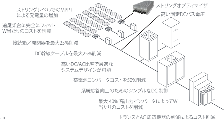
アンプトistring最適化を使用したDC側蓄電池システム
