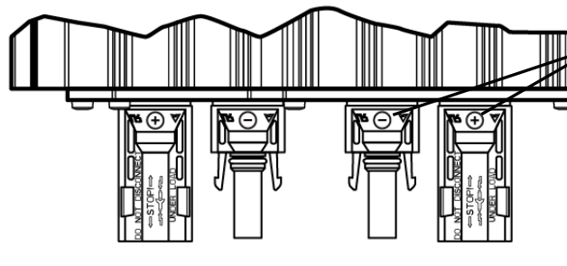
オプティマイザ トップビュー
