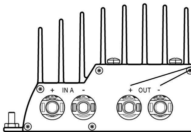
オプティマイザ 正面図
